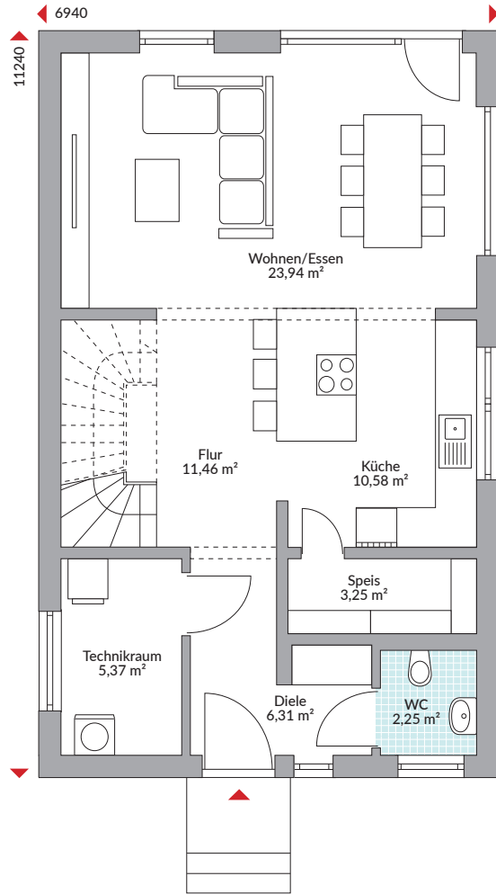
Erdgeschoss 63,16 m 2
