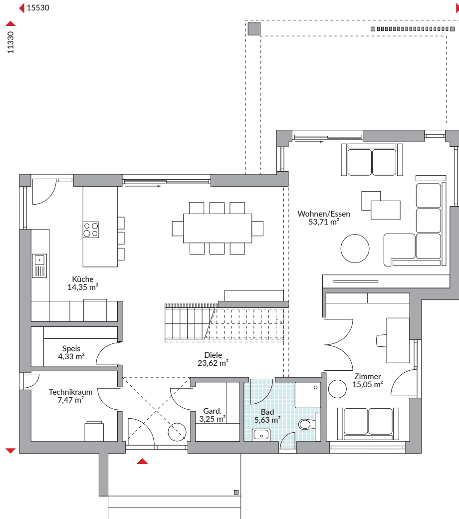
Erdgeschoss 127,41 m 2
