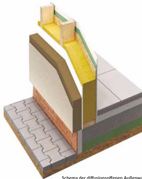
Schema der diffusionsoffenen Außenwand
