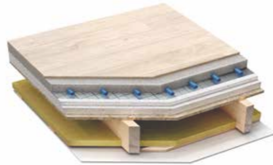
Schema Geschossdecke Erdgeschoss
