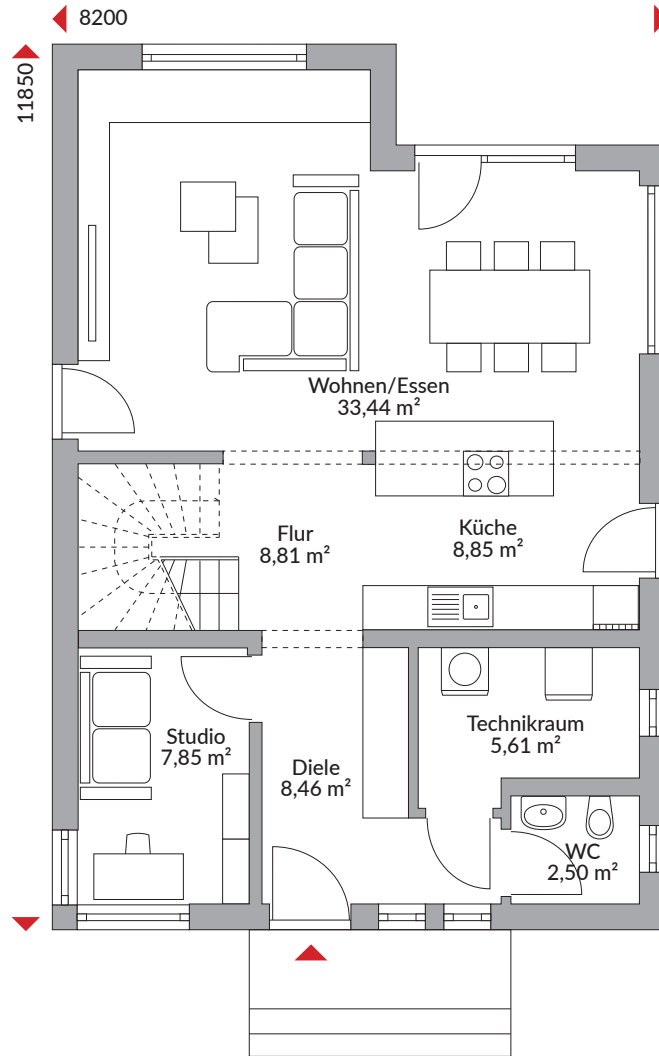
Erdgeschoss 75,52 m 2
