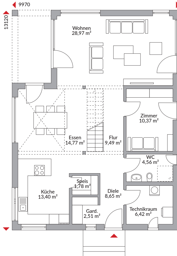
Erdgeschoss 100,92 m 2
