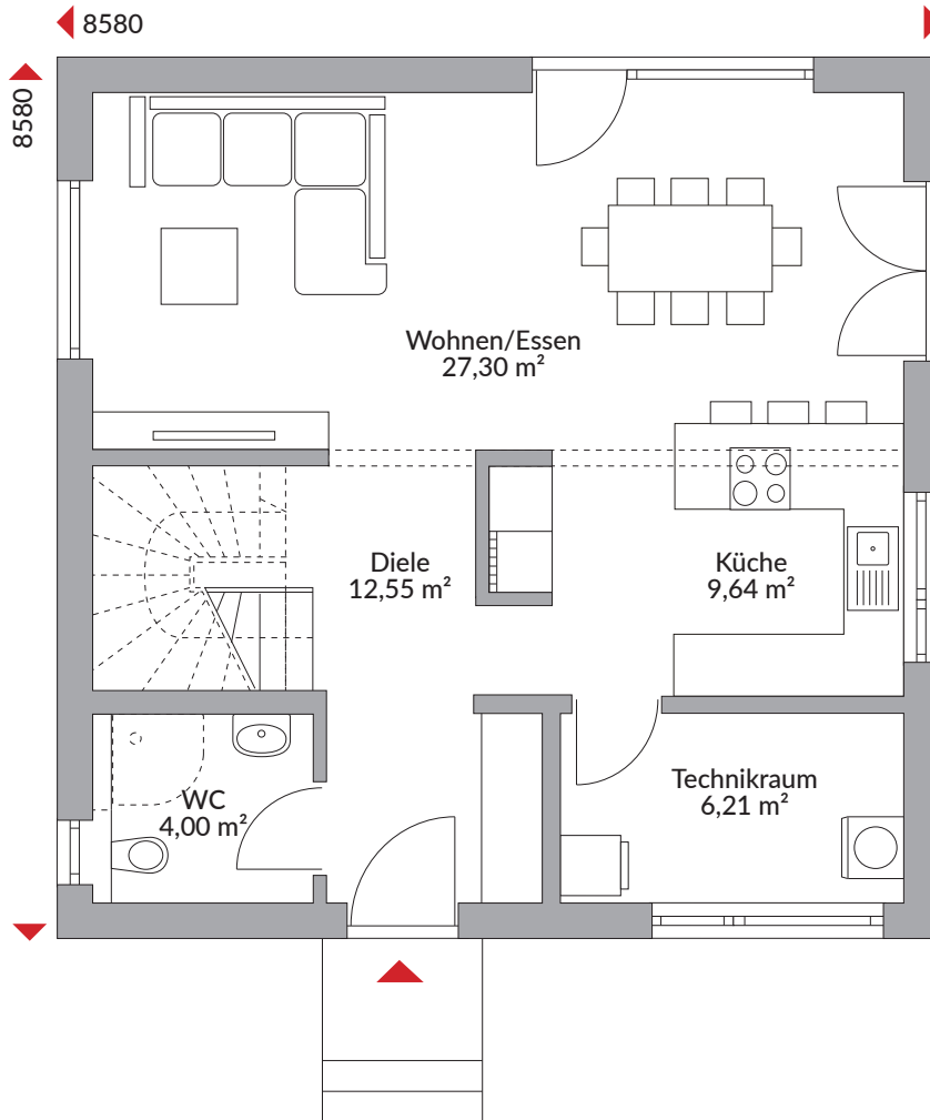
Erdgeschoss 59,70 m 2
