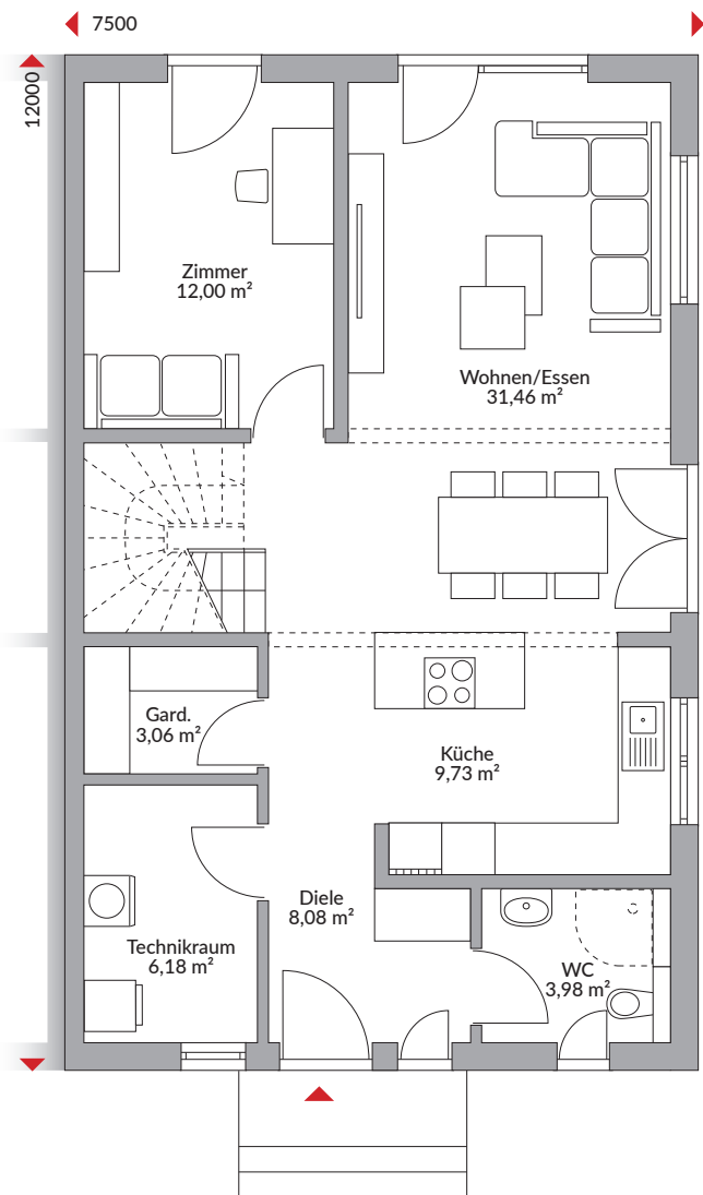
Erdgeschoss 74,49 m 2
