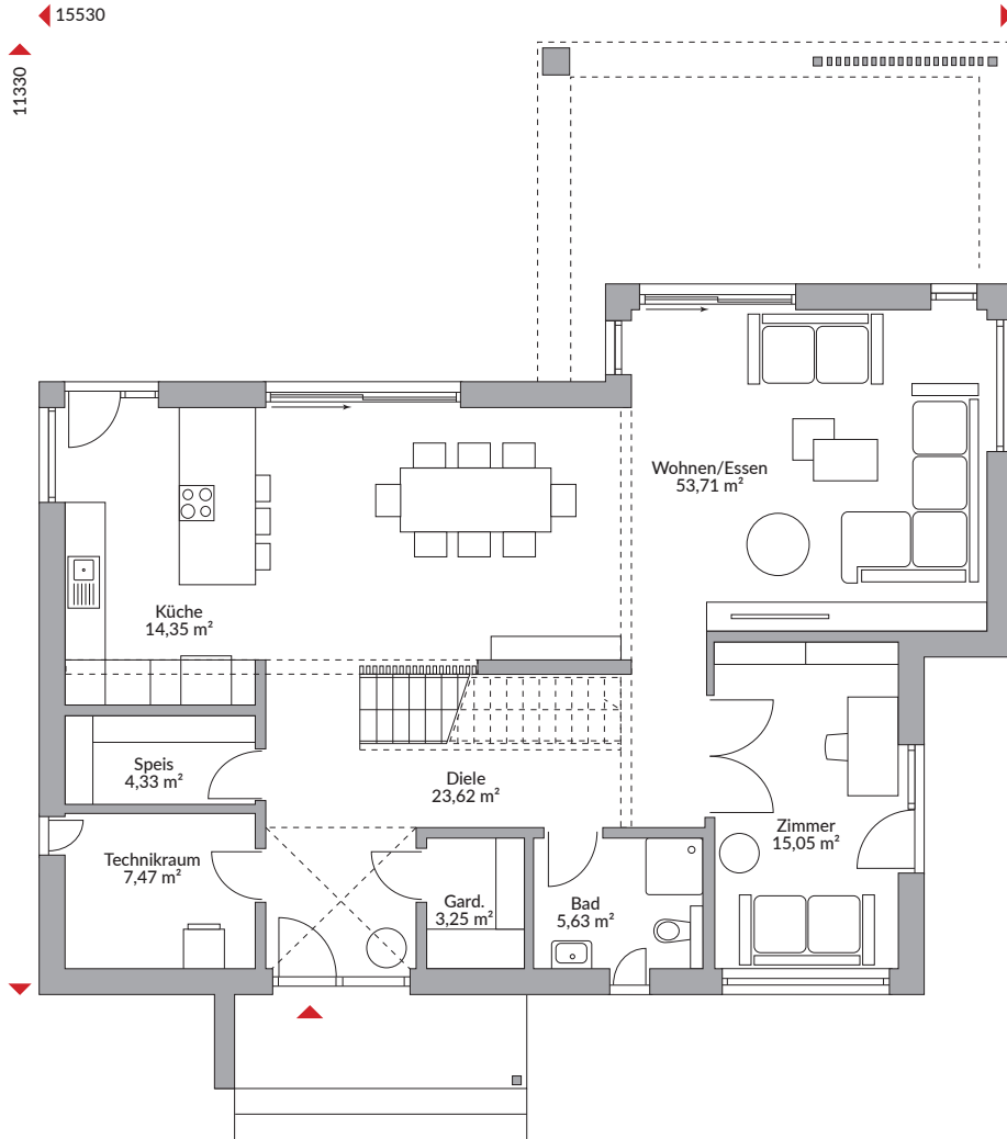
Erdgeschoss 127,41 m 2
