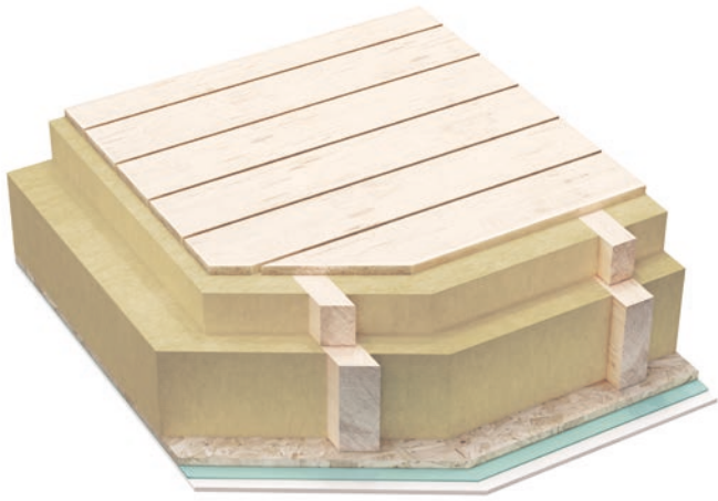
Aufbau der Kehlbalkendecke zum unbeheizten Spitzboden
